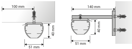
VISTA DI LATO Attacco a soffitto DI SERIE
