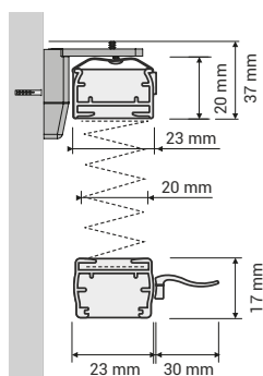
VISTA DI LATO Attacco a parete OPTIONAL
