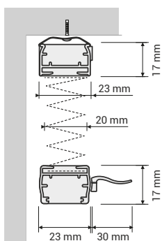
VISTA DI LATO Attacco a soffitto
